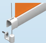
Wandbevestiging
